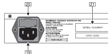
Abb. 3.4: Netzanschluss, Sicherungshalter und Seriennummer
