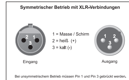
Abb. 8.2: XLR-Stecker
