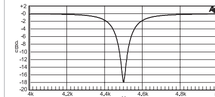
Abb. 4.1: Filterkurve eines sehr schmalbandigen Filters
