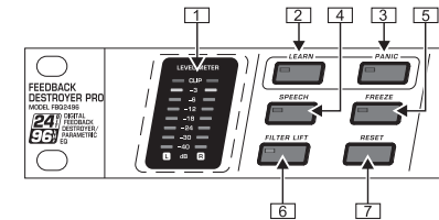
Abb. 3.1: Bedienelemente auf der linken Seite des FBQ2496
