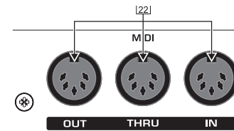
Abb. 3.5: MIDI-Anschluss-Buchsen des FBQ2496
