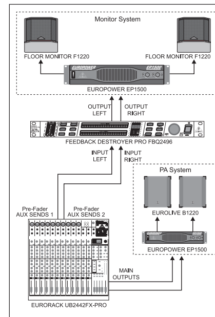
Abb. 5.1: Verwendung des FBQ2496 im Monitorweg
