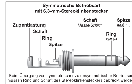
Abb. 8.1: 6,3-mm-Stereoklinkenstecker
