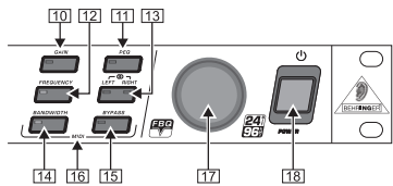
Abb. 3.3: Bedienelemente auf der rechten Seite des FBQ2496
